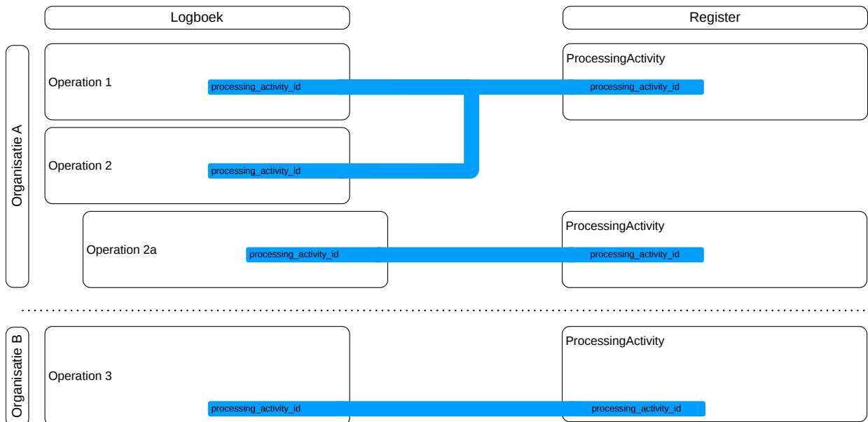
Figuur 7 Afbeelding relaties processing_activity_id tussen Logboek en Register bij meerdere organisaties
