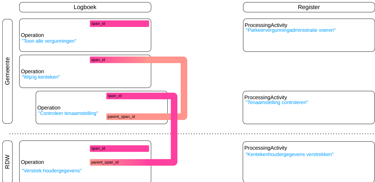
Figuur 16 Afbeelding voorbeeld span_id en parent_span_id bij Gemeente en RDW
