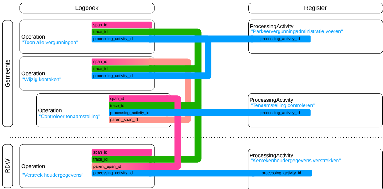
Figuur 17 Afbeelding Voorbeeld met alle span, trace en processing elementen
