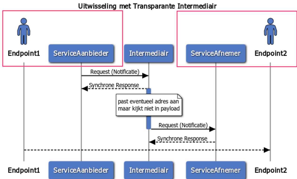
Figuur 12 Transparante Intermediar
