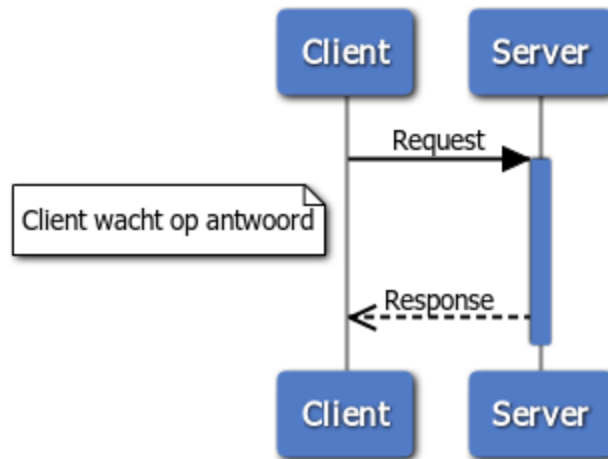
Figuur 10 Synchroon Request
