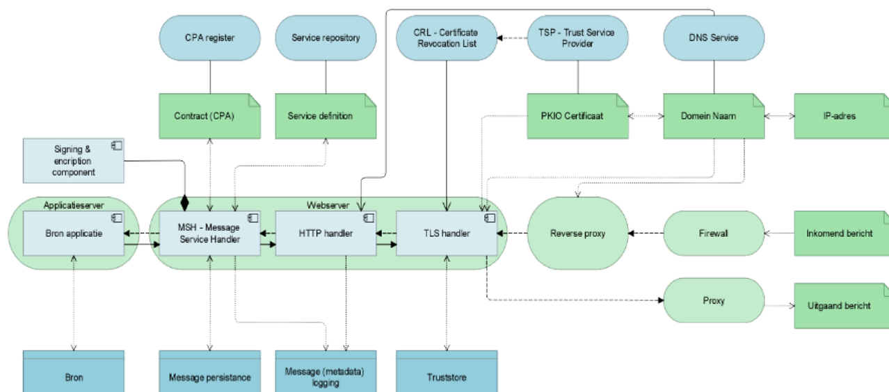
Figuur 9 Referentiemodel gegevensuitwisseling
