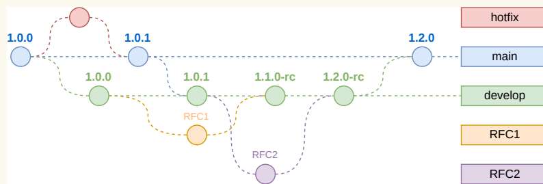
Figuur 8 Gitflow
