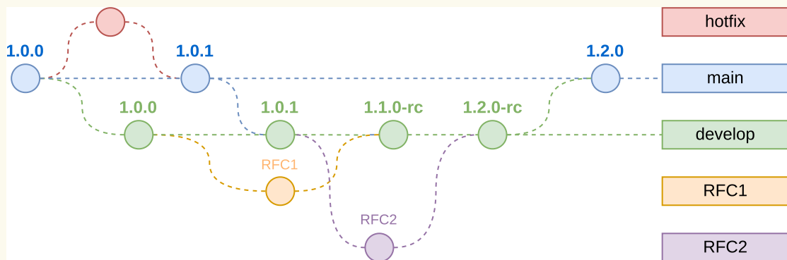
Figuur 6 Gitflow
